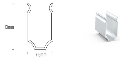
AQS-402-ACC-03 Aluminium Clip
