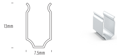
AQS-402-ACC-03 Aluminium Clip
