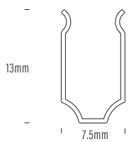
AQS-402-ACC-03 Aluminium Clip
