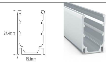
AQS-420-ACC-03 2m Aluminium
