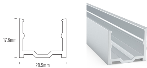
AQS-421-ACC-03 2m Aluminium
