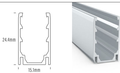
AQS-420-ACC-01 1m Aluminium
